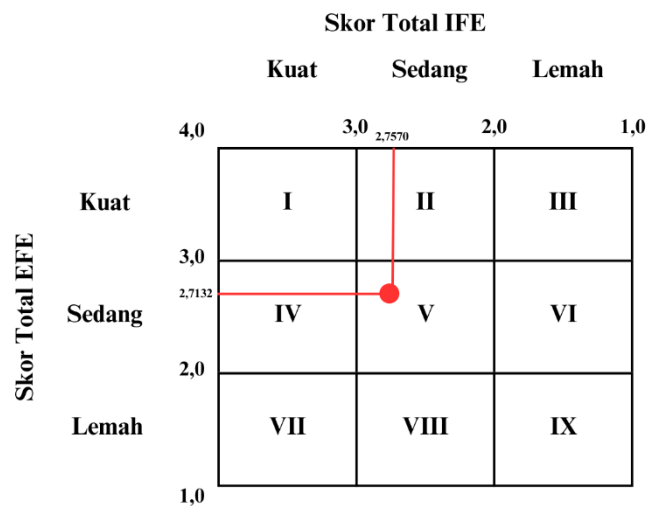
GAMBAR11 Matriks Ie
