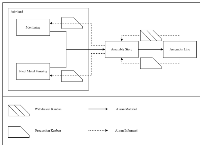
Gambar 7 Mekanisme Kanban
