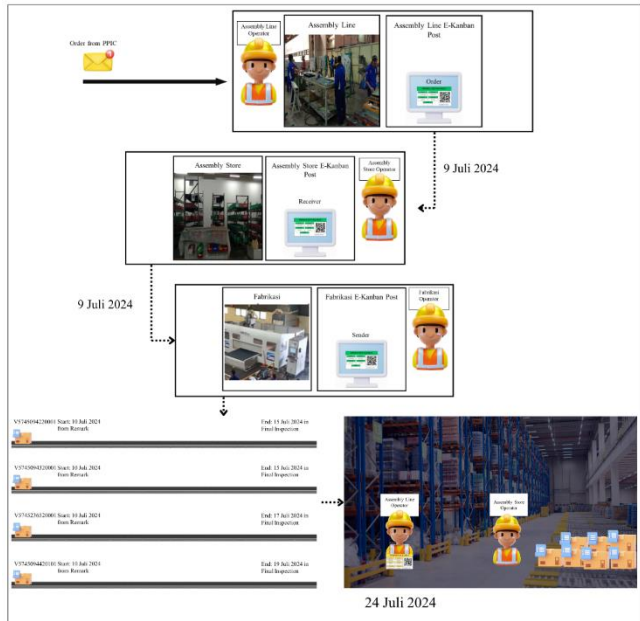
Gambar 24 Skenario Simulasi
