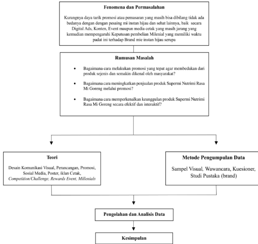
Gambar 1.6 Kerangka Penelitian
