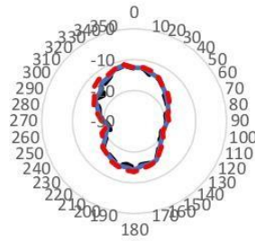
GAMBAR 18. Polarisasi Katun 3.5GHz
