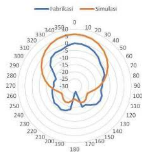
GAMBAR 20. Polaradiasi Azimuth Perban 3.5GHz
