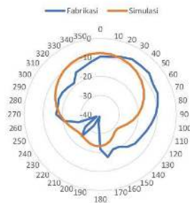
GAMBAR 22. Polaradiasi Azimuth Perban 1.8GHz
