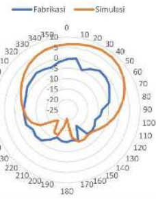
GAMBAR 21. Polaradiasi Elevasi Perban 3.5GHz
