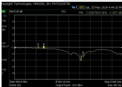
GAMBAR 6. S11 Perban 3.5GHz
