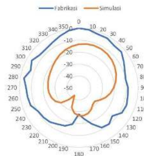
GAMBAR 23. Polaradiasi Elevasi Perban 1.8GHz
