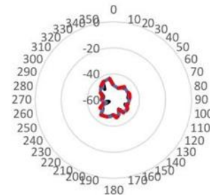
GAMBAR 17. Polarisasi Perban 1.8GHz
