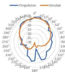
GAMBAR 24. Polaradiasi Azimuth Katun 3.5GHz
