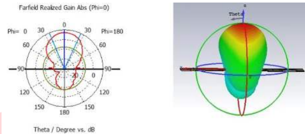
GAMBAR 11 (POLA RADIASI ANTENA ELEVASI PADA THETA DAN PHI)
