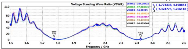
GAMBAR 4 (GRAFIK NILAI VSWR ANTENA SUSUNAN 2 ELEMEN)
