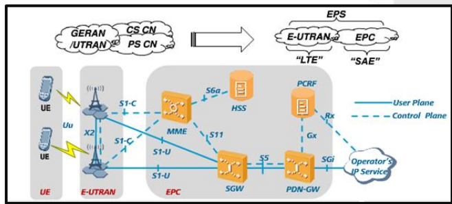
Gambar 1. Arsitektur LTE
