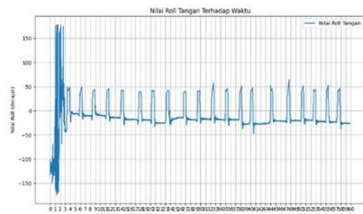
GAMBAR 2 (Grafik Sudut Tangan)
