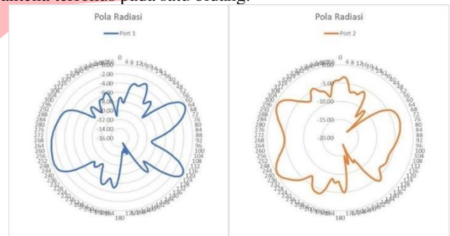
GAMBAR 5 Pola Radiasi
