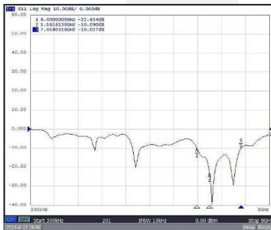
GAMBAR 3 S11 Parameter Pengukuran
