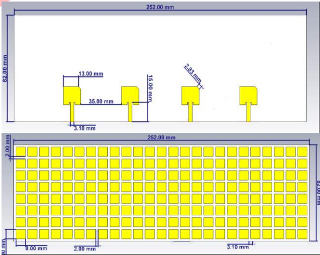
Gambar 1 Antena MIMO 4X4
