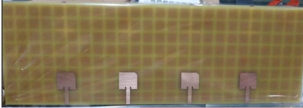
GAMBAR 2 Antena Fabrikasi
