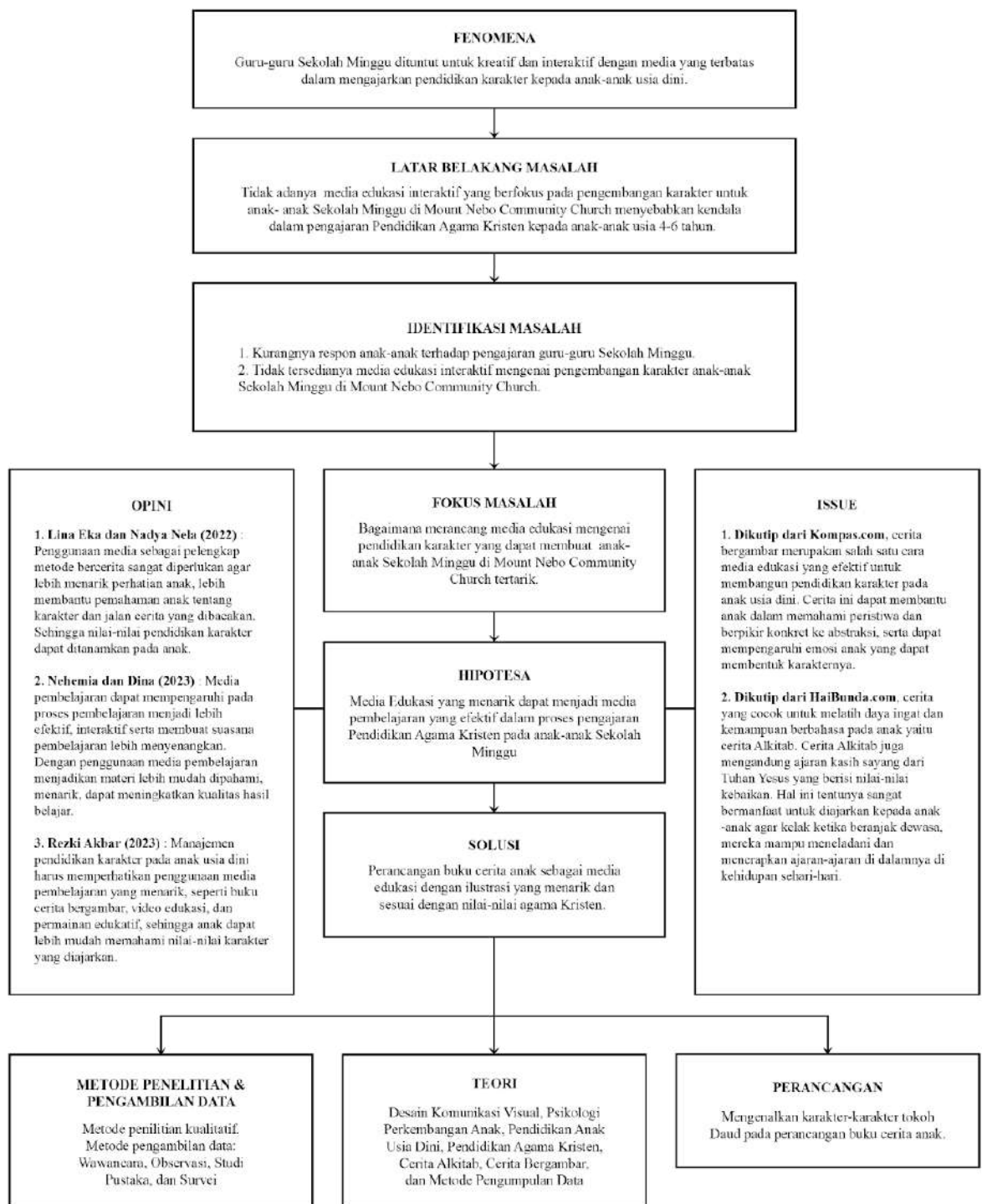
Gambar 1.8.1 Kerangka Penelitian
