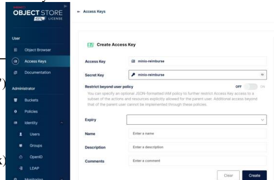
Gambar 3. 7 Pembuatan Access Key
