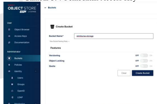
GAMBAR 3. 8 Pembuatan Bucket MinIO
