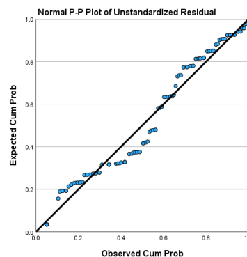
Gambar 4.1 Grafik Uji Normalitas (P-Plot)
