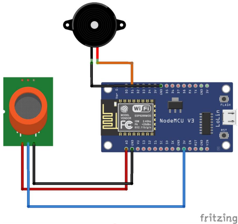
Gambar 9 Skema Rangkaian Sensor
