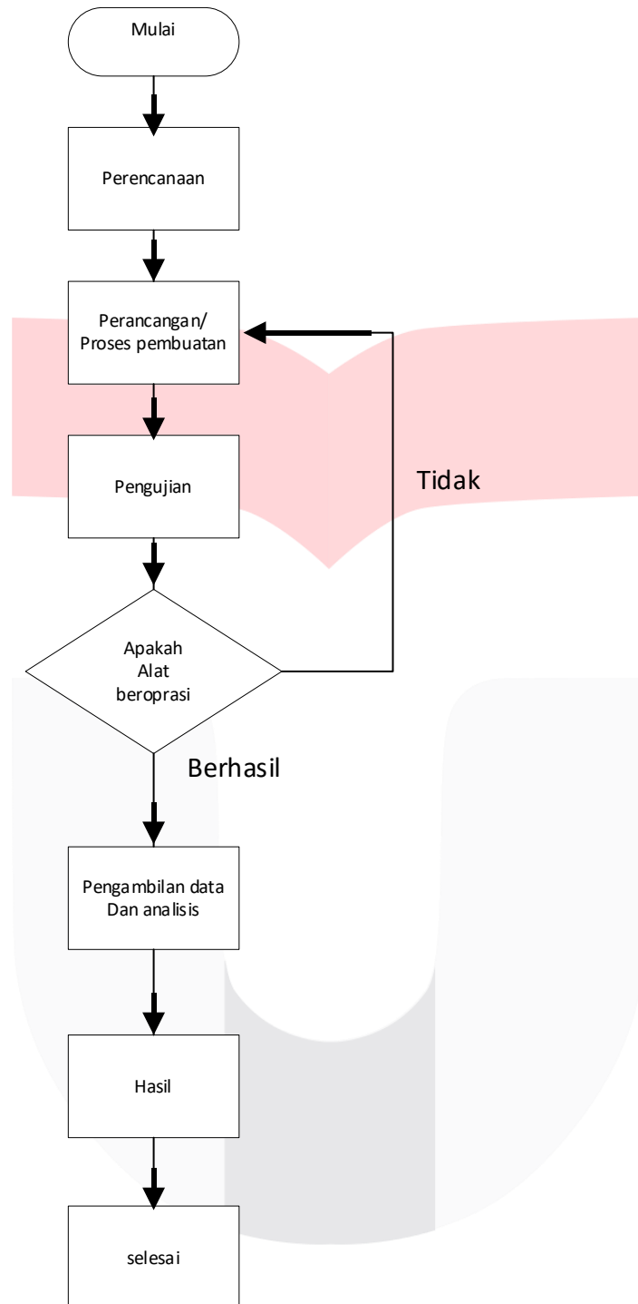
Gambar 7 Alur Perancangan
