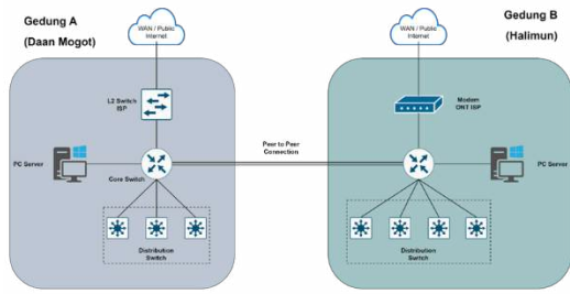
Gambar 2 (Desain Jaringan Eksisting)
