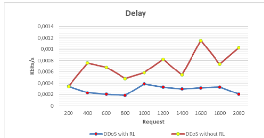
GAMBAR 4.3 Grafik Delay
