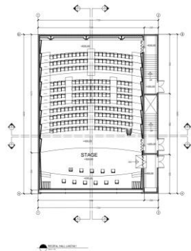
Gambar 13 Layout lantai dasar Sumber: dokumentasi penulis
