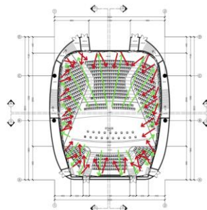
Gambar 7 Skema pemantulan suara pada dinding
