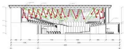
Gambar 6 Skema pemantulan suara pada plafon Sumber: dokumentasi penulis
