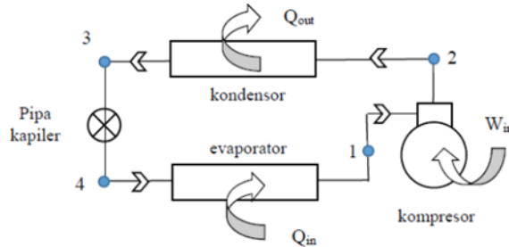
Gambar 1. Siklus Refrigerasi
