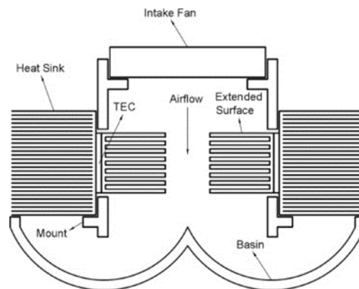
Gambar 3. Atmospheric Water Generator menggunakan Peltier Effect
