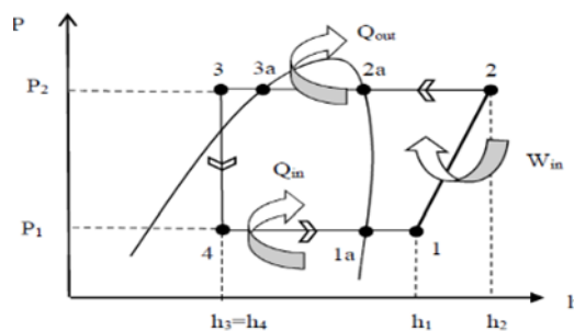
Gambar 2. Siklus Kompresi Uap
