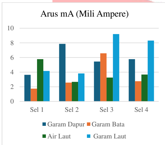
GAMBAR 4. 5 Grafik Arus
