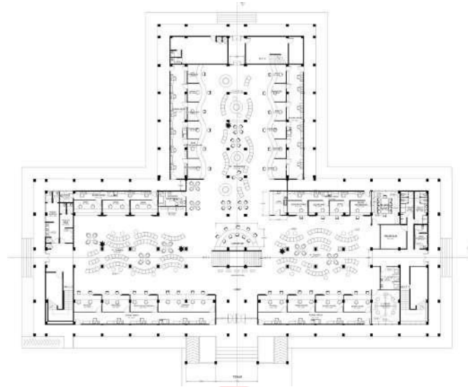
Gambar 7. Layout Perancangan
