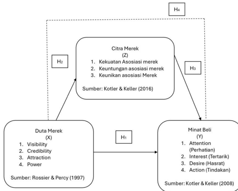
Gambar 2.1 Kerangka Pemikiran
