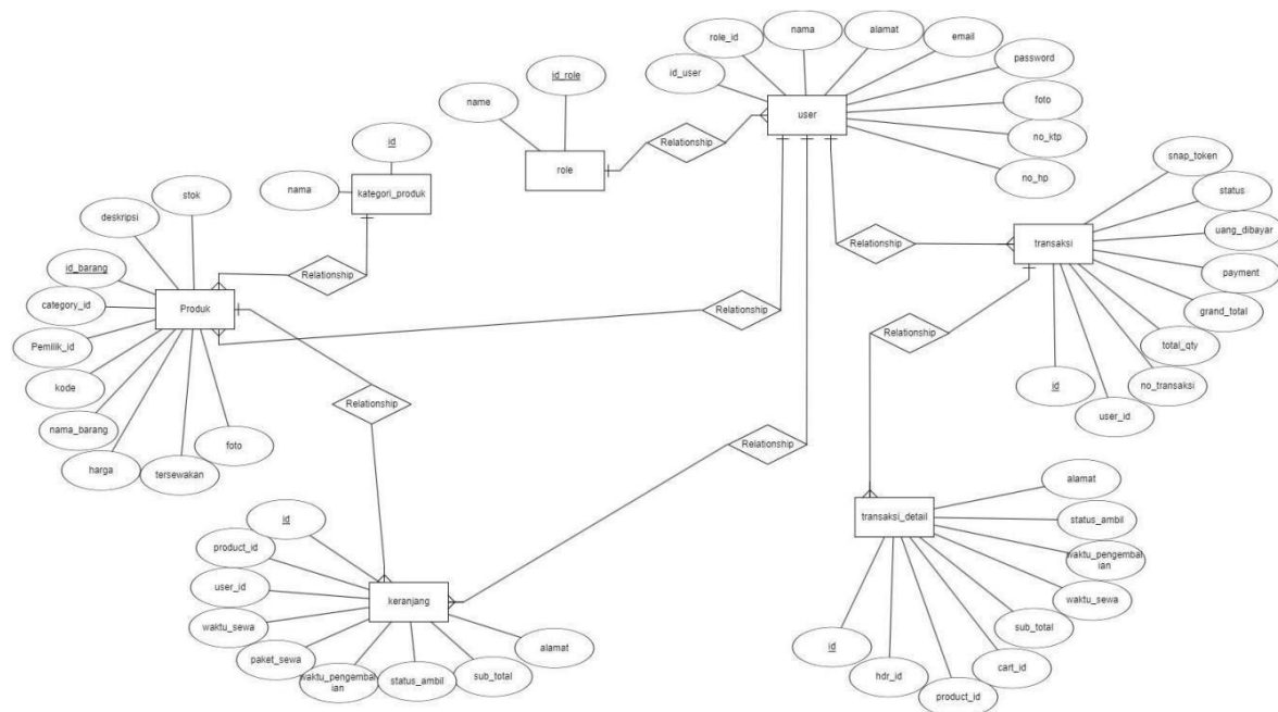
Gambar 14. ERDPlus
