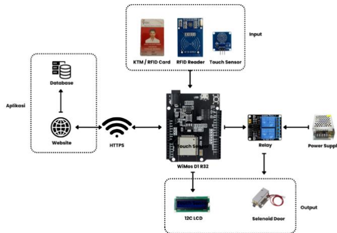
Gambar 3. 3. 1. 1. Perancangan Prototype
