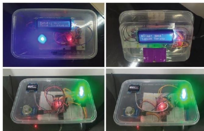
Gambar 4. 7 Perangkat Deteksi Api
