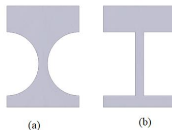
Gambar I.3 Tipe flexure hinge , (a) Notch Hinge , (b) leaf spring hinge (Dimodifikasi, dengan izin dari Ling dkk., (2023), © Elsevier)
