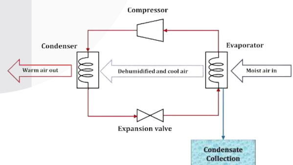
Gambar 1 Atmospheric Water Generator menggunakan sistem kompresi uap[2]
