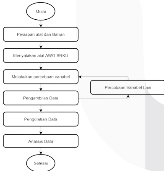
GAMBAR 3. Skenario pengujian
