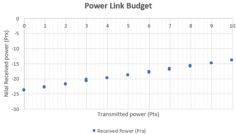
Gambar 3 Grafik Hasim Simulasi Power Link Budget
