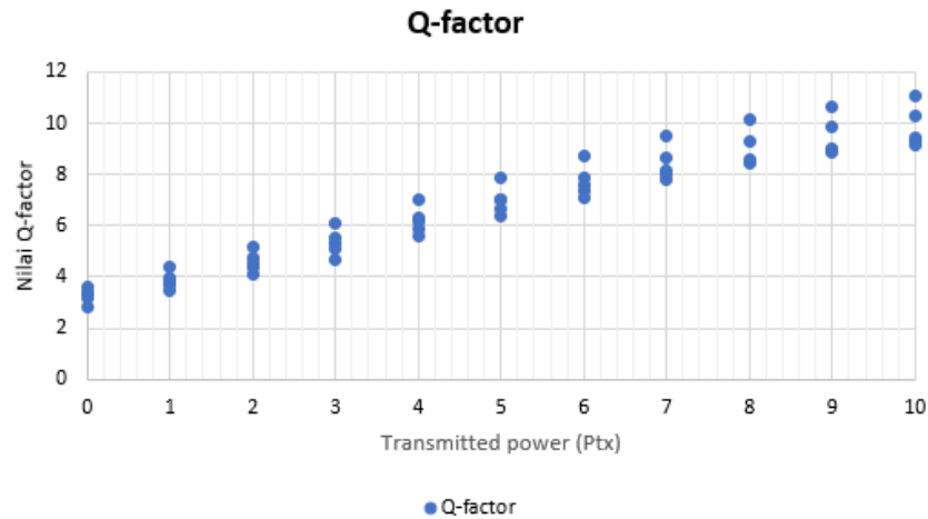
Gambar 5 Grafik Hasil Simulasi Nilai Q -factor
