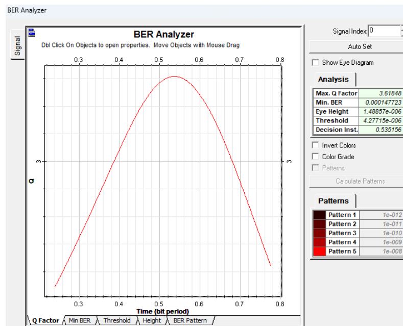
Gambar 9 Hasil BER dan Q-factor Terburuk Pada Link Backhaul
