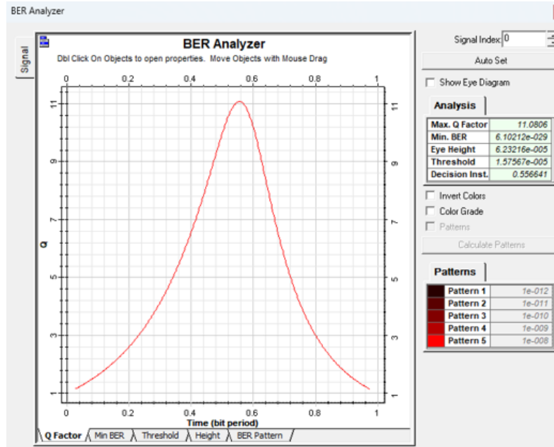
Gambar 7 Hasil BER dan Q-factor Terbaik Pada Link Backhaul
