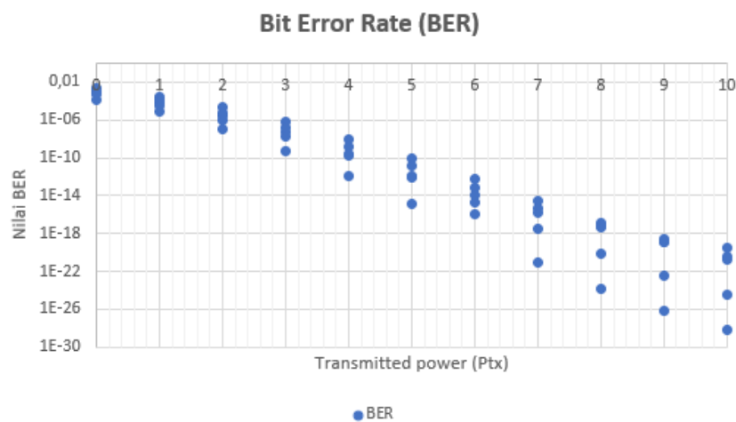
Gambar 6 Grafik Hasil Simulasi Nilai BER
