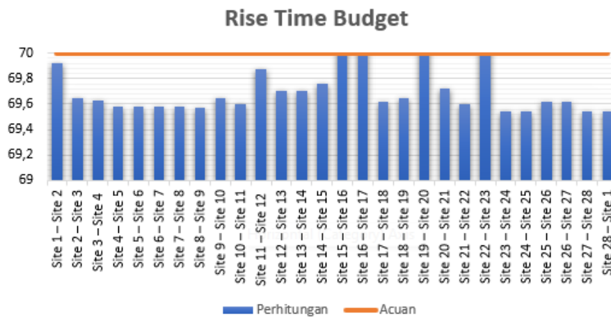
Gambar 4 Grafik Perbandingan Nilai Rise Time Budget
