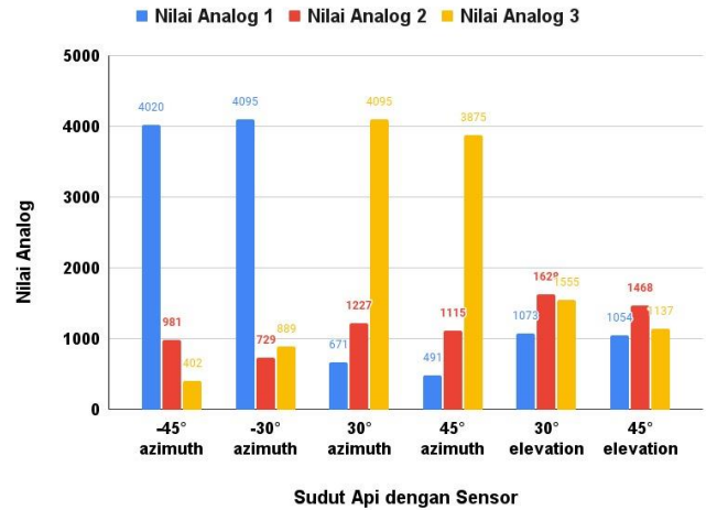
Gambar 4. Hasil Pengujian Sensor IR Flame dengan Azimuth dan Elevasi
