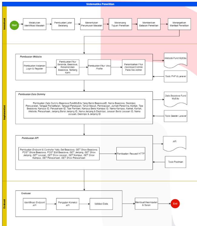
Gambar 3 Sistematika Penelitian
