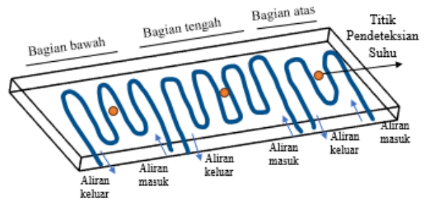
Gambar 7 Desain 2 Pendistribusian Cairan
