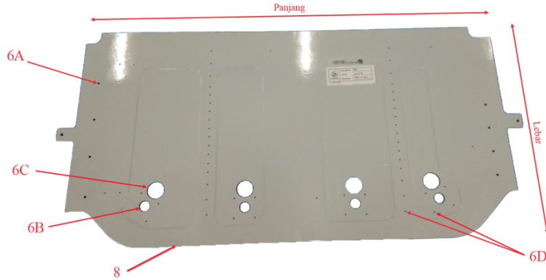
Gambar I.1 Komponen Panel 3 Fuel Lower bagian atas dengan nomor CTQ (Sumber : Dokumen Perusahaan)
