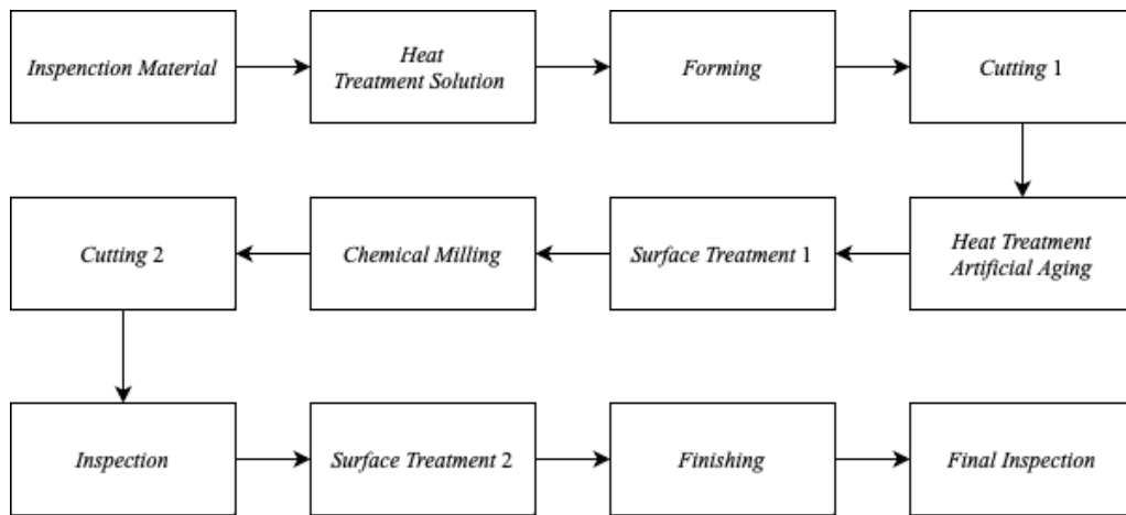
Gambar I.3 Alur proses produksi komponen panel 3 fuel lower (Sumber: Dokumen Perusahaan)
