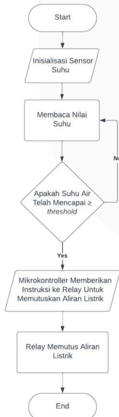
GAMBAR 5. Flowchart Sistem Pengendali Aliran Listrik
