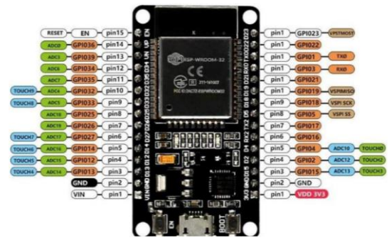
GAMBAR 3. Mikrokontroler ESP32
