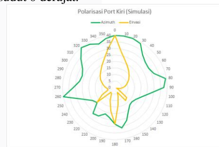
GAMBAR 20 Perbandingan Polarisasi Azimuth dan Elevasi Port Kiri
