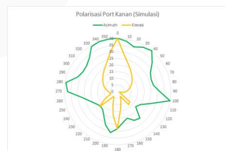
GAMBAR 21 Perbandingan Polarisasi Azimuth dan Elevasi Port Kanan
