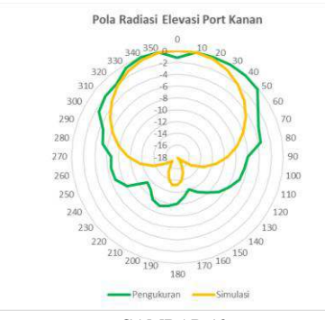
GAMBAR 19 Perbandingan Pola Radiasi Elevasi Port Kanan
