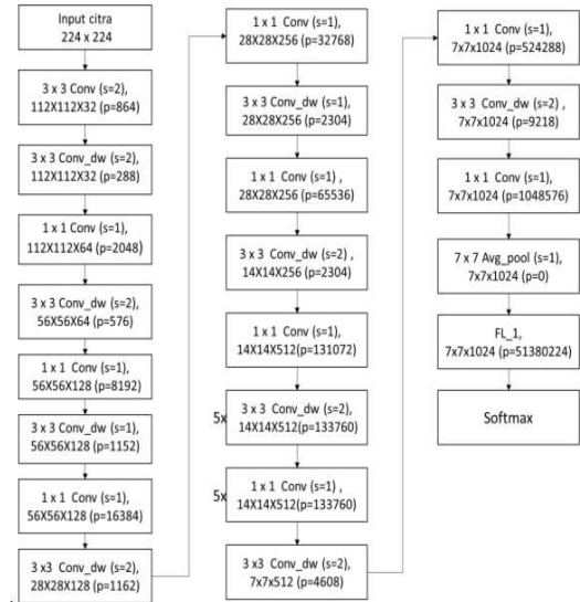
GAMBAR 9 Arsitektur mobilenet
