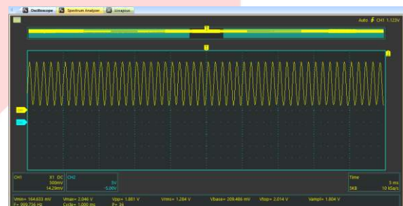
GAMBAR 7 Pengujian 1000 Hz pada tampilan Osiloskop
