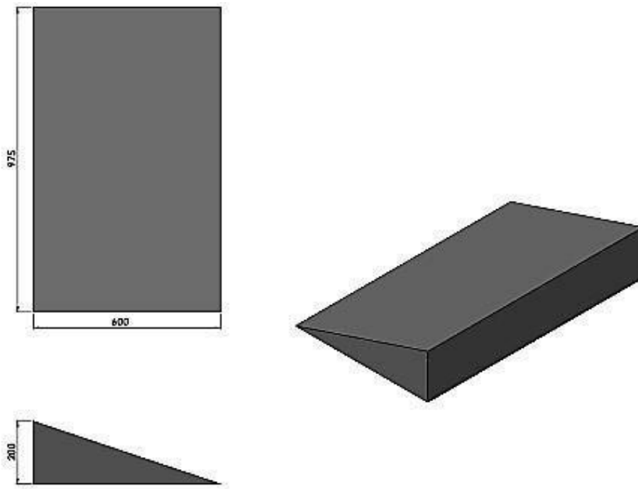
Gambar 1.7 Rintangan Bidang Miring (dimensi dalam mm)
