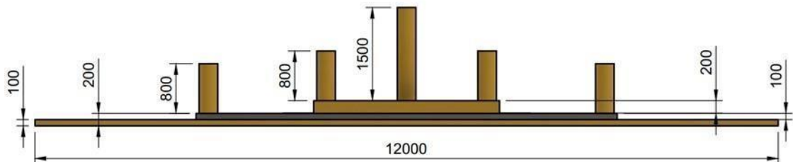
Gambar1.4 Tinggi dari setiap area dan tiang pada lapangan permainan
