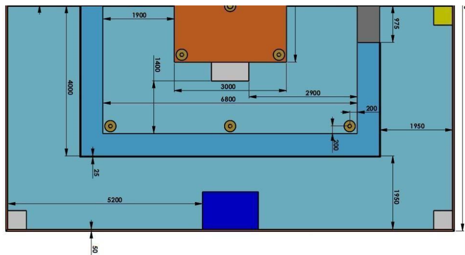
Gambar 1.6 Rintangan pada Blue/Red Area
