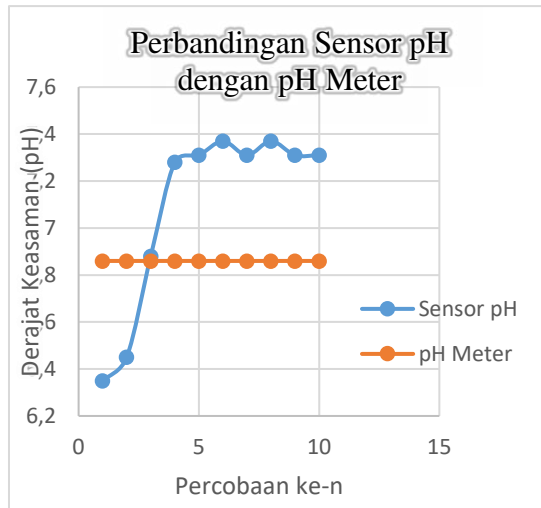
GAMBAR 4.3 Penguian Sensor pH 6,86
