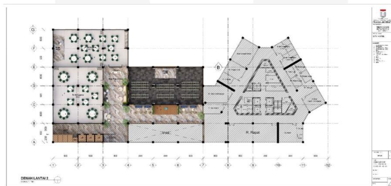
Gambar 4. 2 Layout Lantai 2 Sumber: (Analisis Pribadi, 2023)
