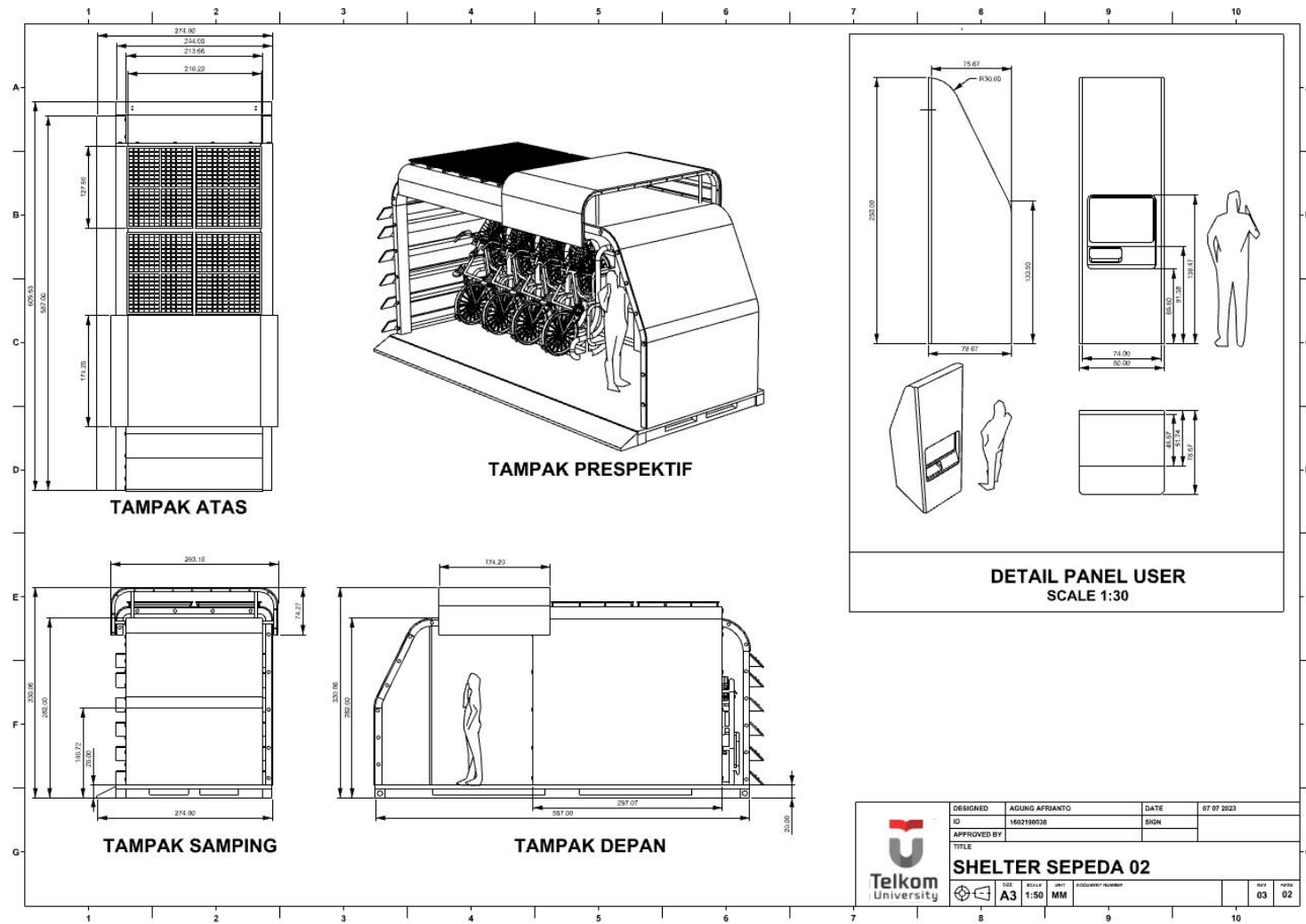
Lampiran 1. 2. Gambar Teknik Fasilitas Selter Sepeda Model 2 Sumber : Dokumen Pribadi (2023)
