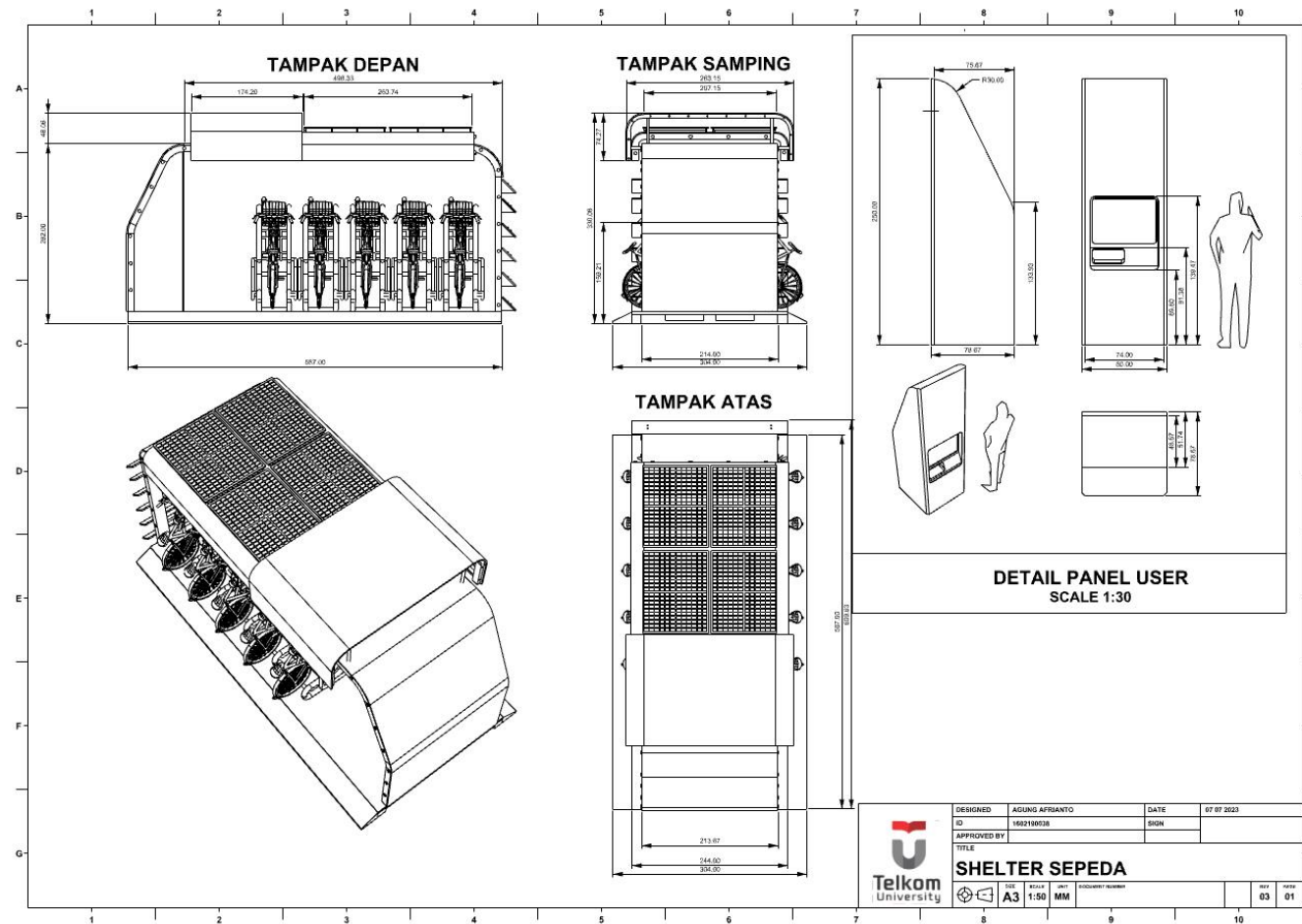
Lampiran 1. 1. Gambar Teknik Fasilitas Selter Model 1 Sumber : Dokumen Pribadi (2023)
