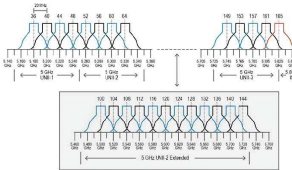
GAMBAR 1 Frekuensi 5 GHz [3]
