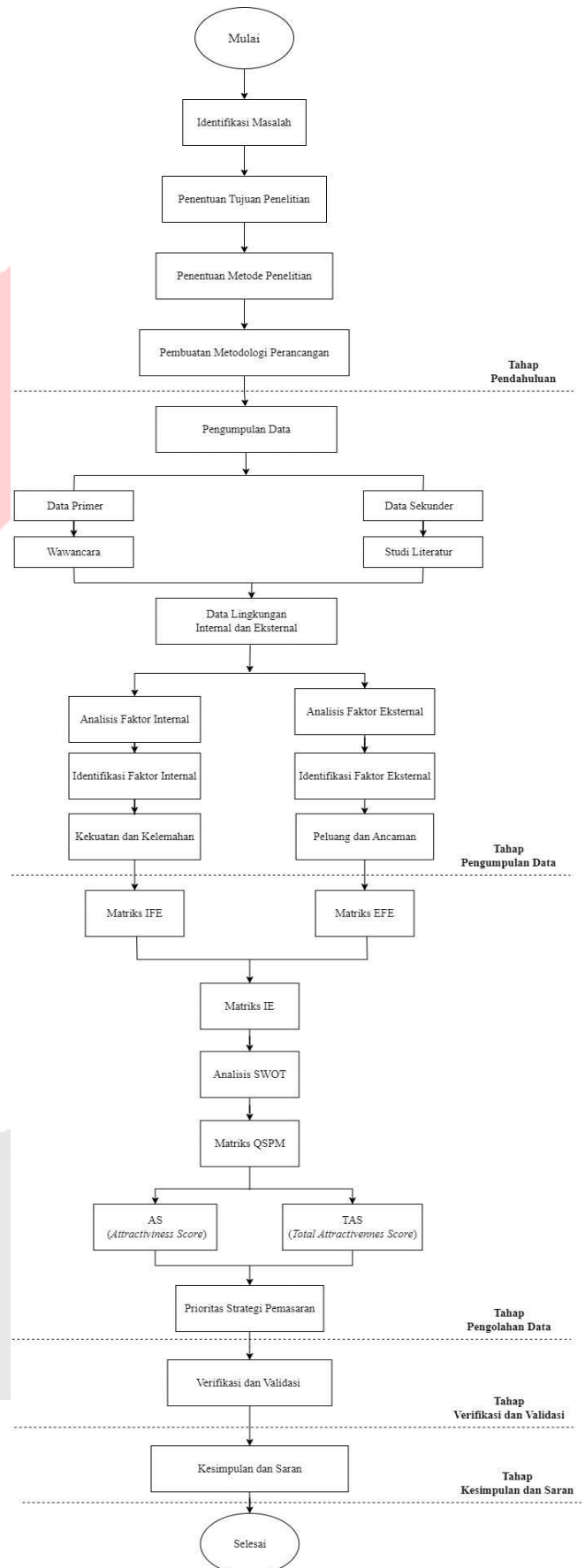
GAMBAR 5 (Sistematika Perancangan)
