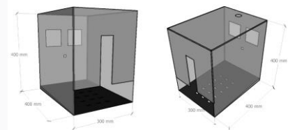
GAMBAR 1 Desain kandang
