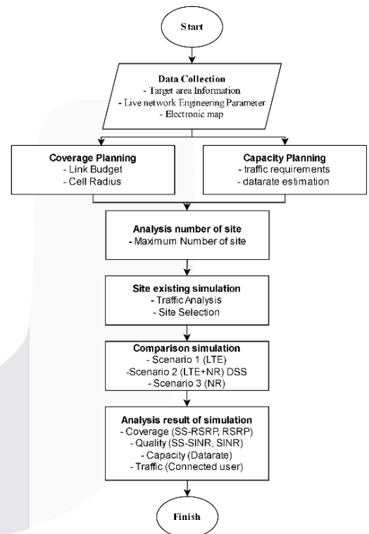
GAMBAR 3.2 Diagram alir perancangan 5G NR.
