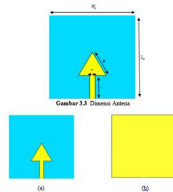
Gambar 3.4 (a) Tampak Depan dan (b) Tampak Belakang dari Antena
