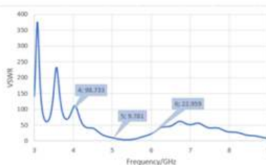
Gambar 3.6 Grafik VSWR Antena sebelum optimasi
