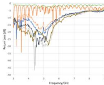
Gambar 3.13 Pengaruh Jarak Antena pada phantom
