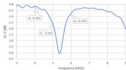
Gambar 3.5 Grafik Return Loss Antena Sebelum dioptimasi
