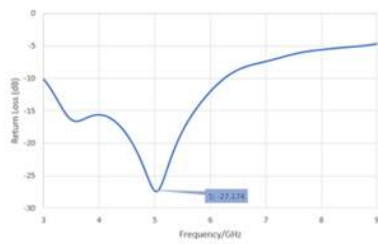
Gambar 3.9 Grafik Return Loss Antena Optimasi
