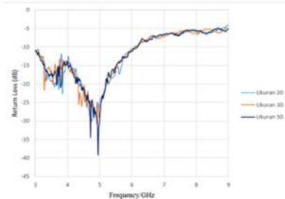
Gambar 3.15 Grafik Return Loss Phantom Kepala dengan Kanker
