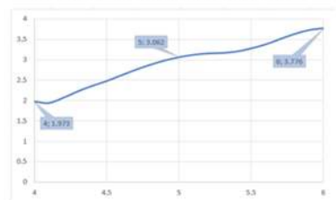
Gambar 3.11 Grafik Gain Antena Optimasi
