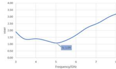
Gambar 3.10 Grafik VSWR Antena Optimasi
