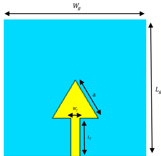
Gambar 3.3 Dimensi Antena
