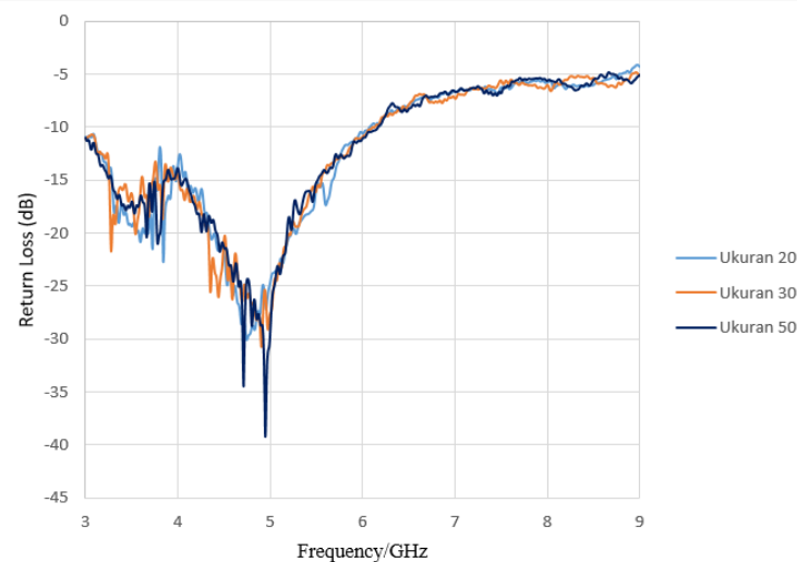
Gambar 3.15 Grafik Return Loss Phantom Kepala dengan Kanker
