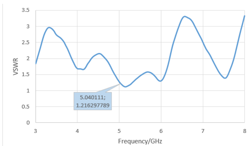
Gambar 4.3 Hasil Pengukuran VSWR
