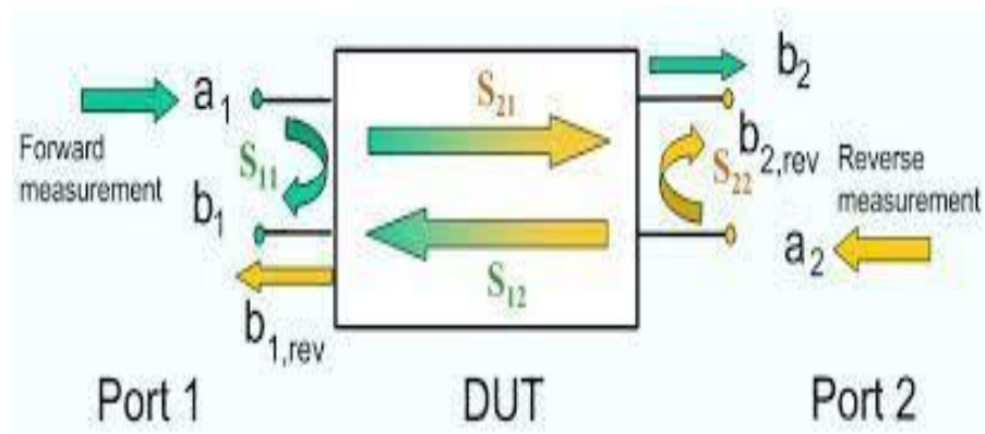
Gambar 2.5 Proses S-Parameter pada port 1 dan port 2
