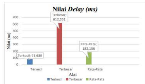
GAMBAR 4.5 Grafik Nilai Delay
