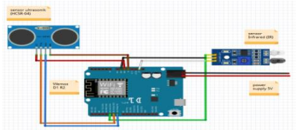
GAMBAR 3.2 Desain Perangkat Keras
