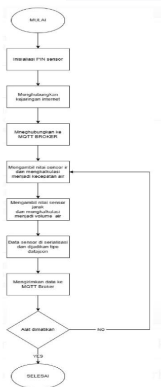
GAMBAR 3.3 Flowchart Perancangan Perangkat Peras
