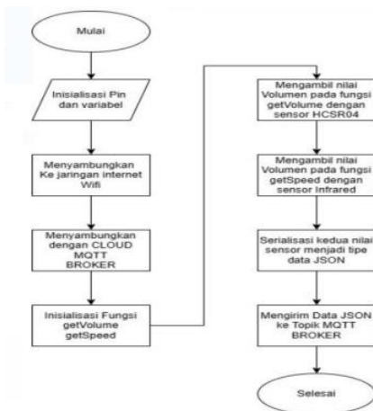
GAMBAR 3.4 Diagram Alir Wemos D1 R2
