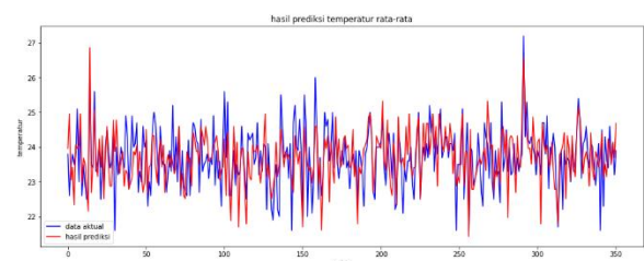
Gambar 3 Data hasil prediksi parameter suhu
