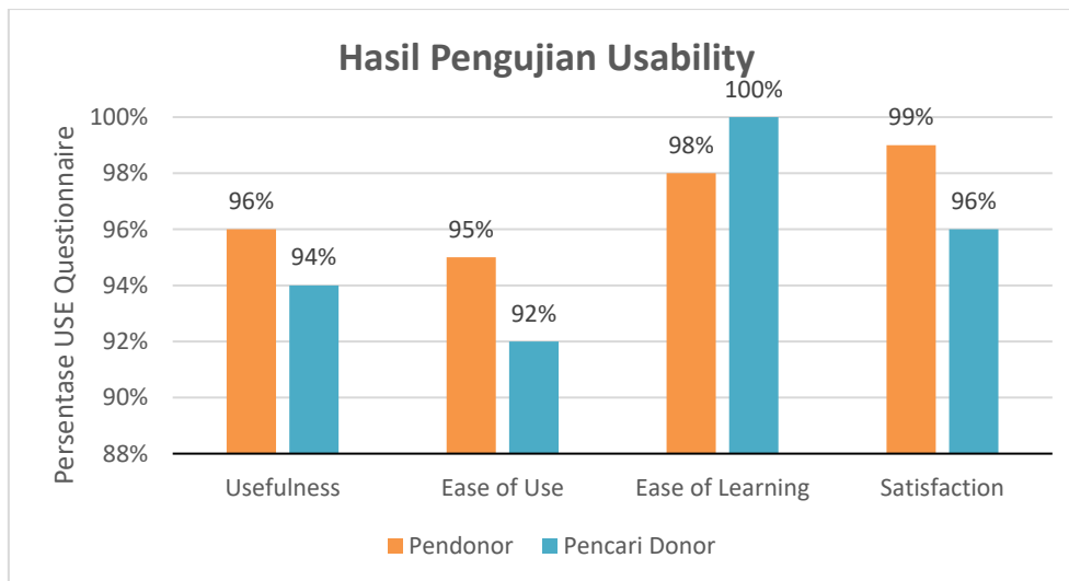
Gambar 2. Hasil pengujian USE Questionnaire
