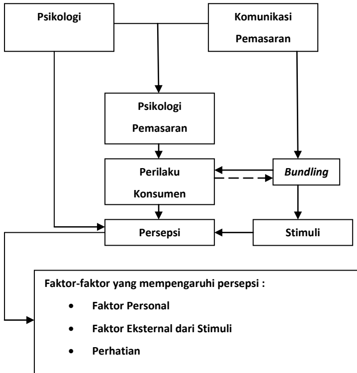
Gambar 2.6 Kerangka Pemikiran
