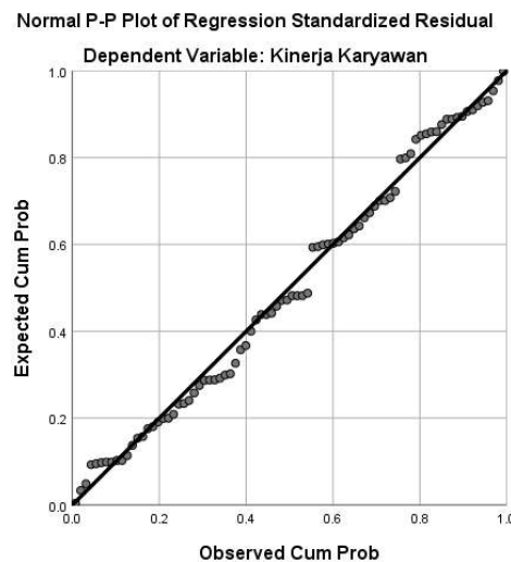
Gambar 3.2 Uji P-Plot
