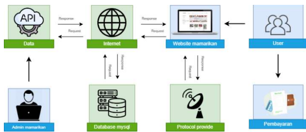
GAMBAR 3 ARSITEKTUR APLIKASI
