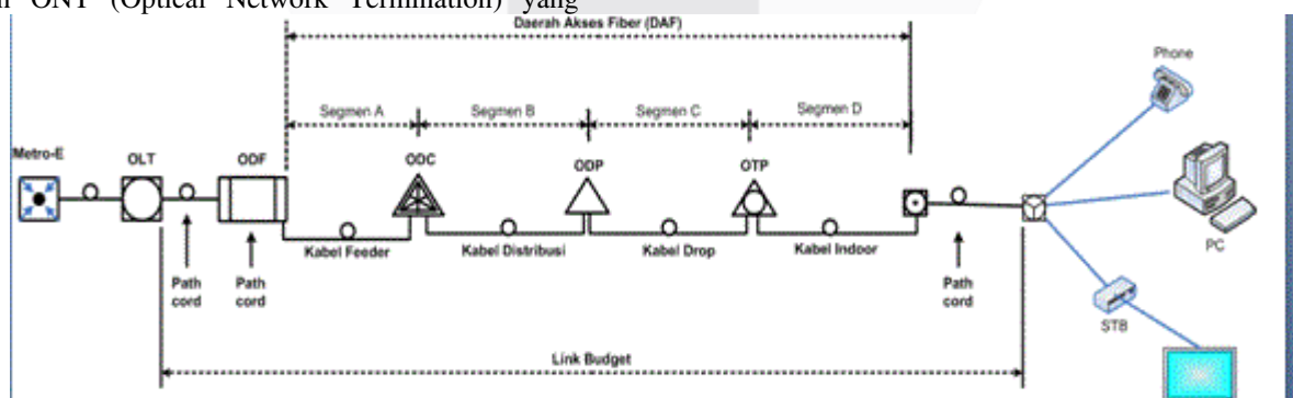
GAMBAR 2.2 GAMBAR JARINGAN FTTH
